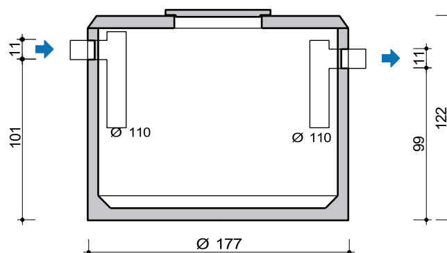
DOORSNEDE COUPE
