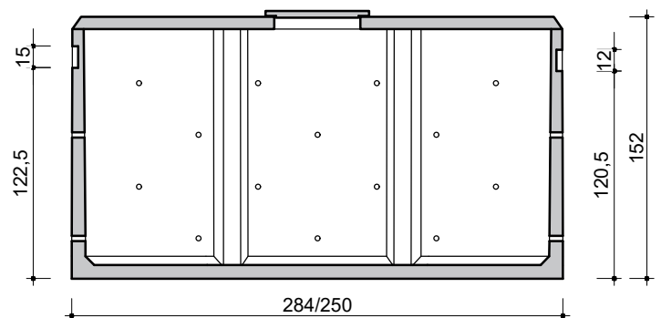
DOORSNEDE COUPE
