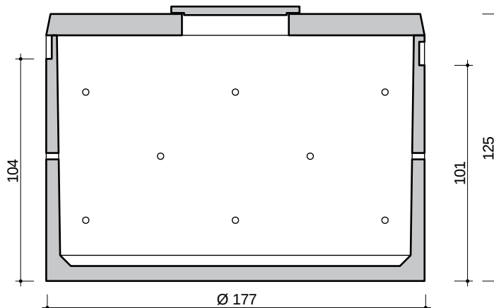
DOORSNEDE COUPE
