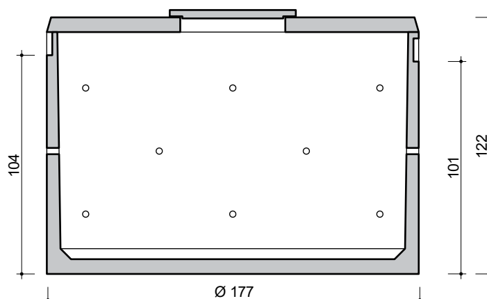
DOORSNEDE COUPE
