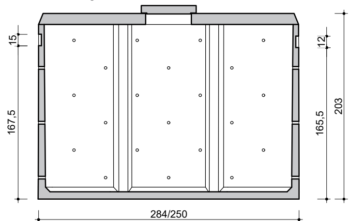
DOORSNEDE COUPE
