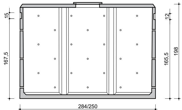
DOORSNEDE COUPE
