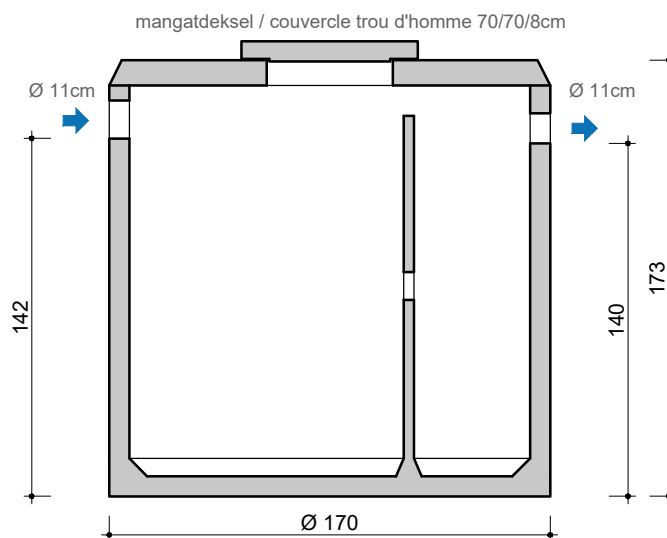
DOORSNEDE COUPE
