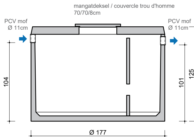
DOORSNEDE COUPE
