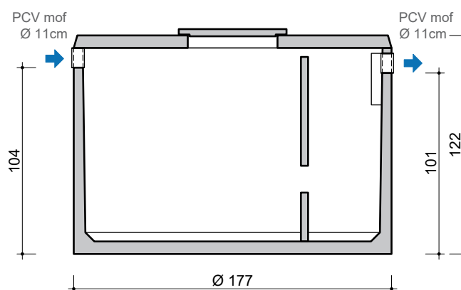
DOORSNEDE COUPE
