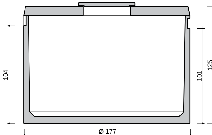
DOORSNEDE COUPE
