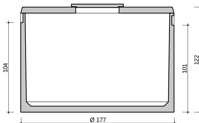
DOORSNEDE COUPE
