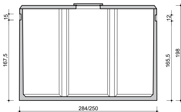
DOORSNEDE COUPE
