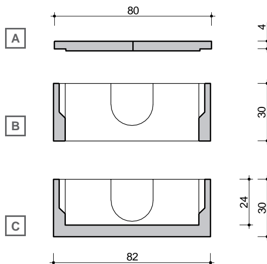
DOORSNEDES COUPES
