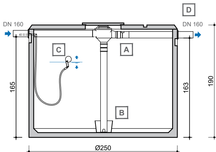
DOORSNEDE COUPE
