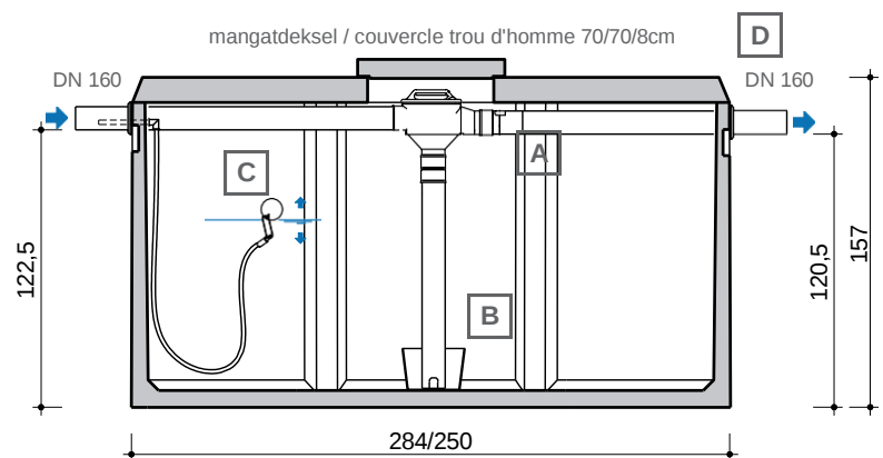
DOORSNEDE COUPE
