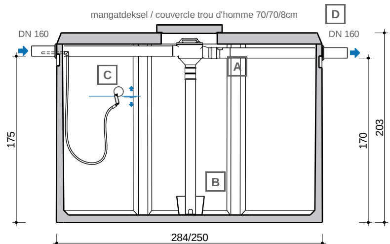
DOORSNEDE COUPE
