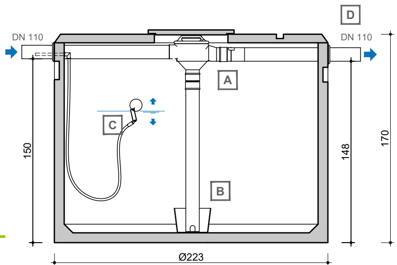
DOORSNEDE COUPE
