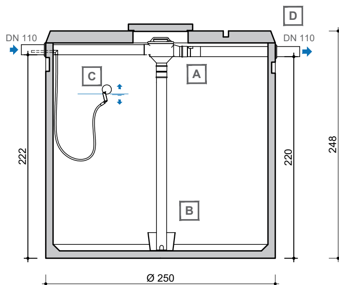
DOORSNEDE COUPE
