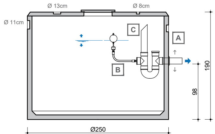
DOORSNEDE COUPE
