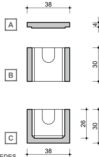
DOORSNEDES COUPES
