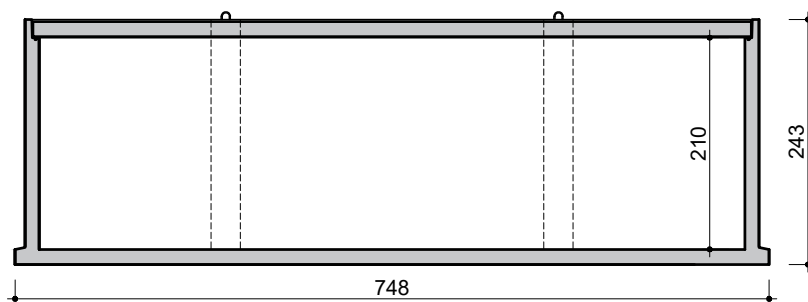
LANGSE DOORSNEDE COUPE LONGITUDINALE
